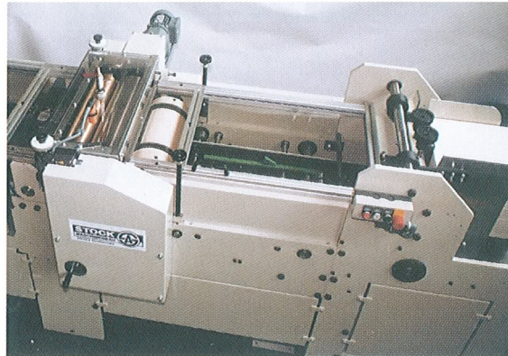
Trägerbogen-Anleger mit Fasson-Leimwerk Substrate sheet feeder with stencil gluing unit
